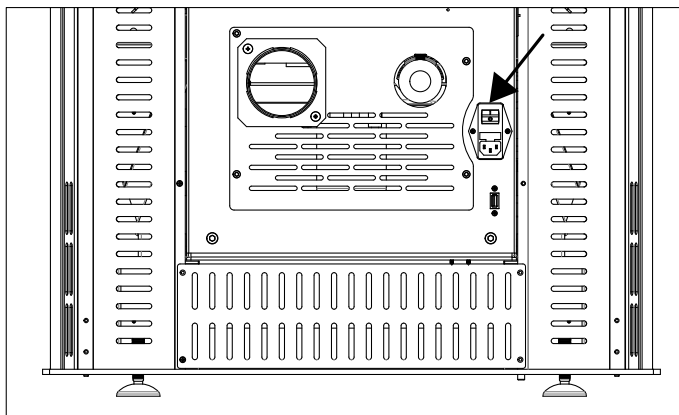
COLLEGAMENTO ELETTRICO DELLA STUFA
