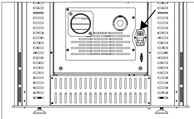
BRANCHEMENT ÉLECTRIQUE DU POËLE
